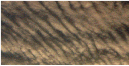
Cirrocumulus
