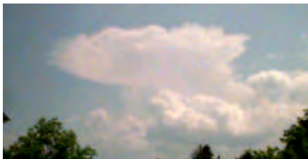
Cumulonimbus
