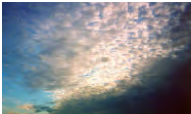
Altocumulus
